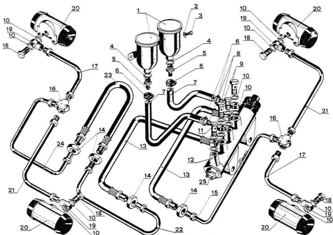
Tav. 09 Impianto Frenatura
