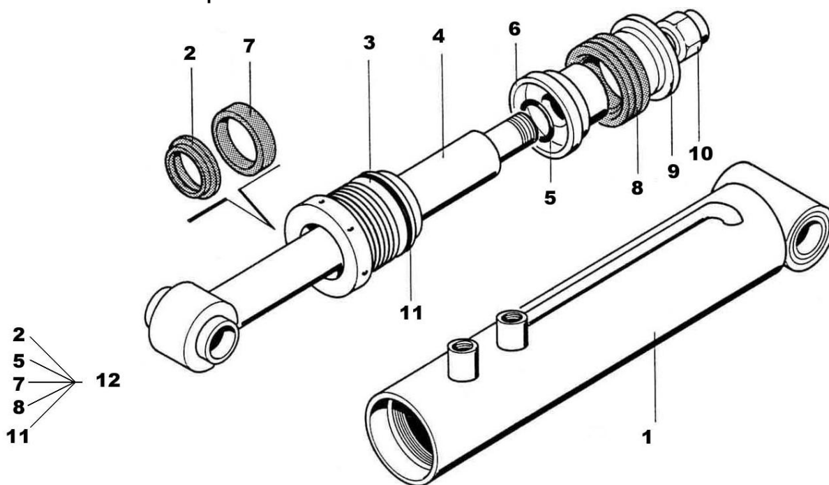
Tav. 11 Cilindro sollevamento benna Tav. 14 Cilindro rotazione pala
